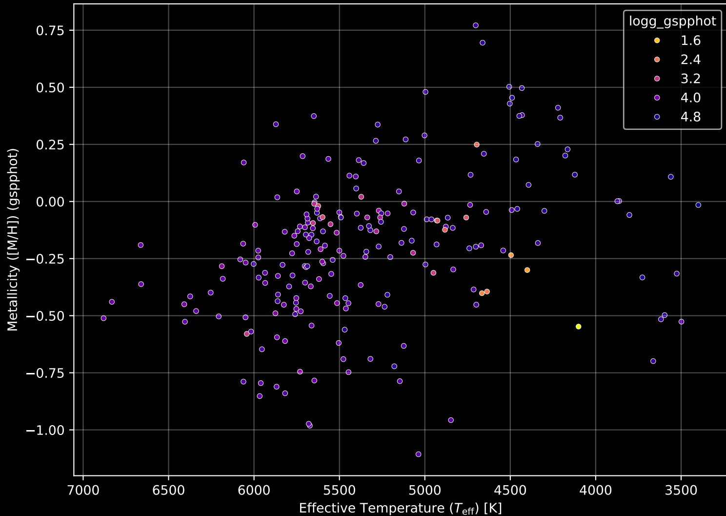
APOGEE DR17 Field: [134-51-O] Stellar Population Parameters (n= 216)
